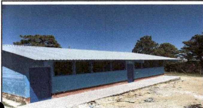
Foto1: Finalización de sustitución de lamina por lamina aluzinc calibre 26
